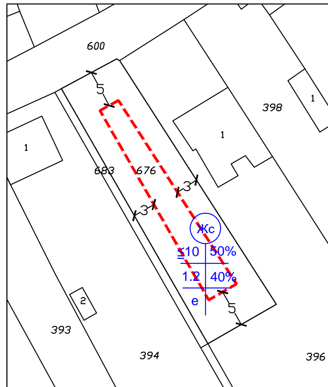
ИЗРАБОТВАНЕ НА ПУП - ПЗ ЗА ПОЗЕМЛЕН ИМОТ №72624.905.676 ПО КК НА ГР. ДОБРИЧ, М-СТ "ГААЗИ БАБА", ОБЩ. ГРАД ДОБРИЧ, ОБЛ. ДОБРИЧ
